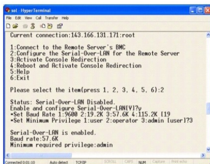
図 3-20 SOL 設定、例 3
