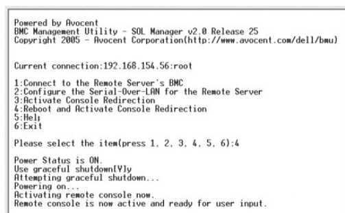
図 3-22 再起動の例
